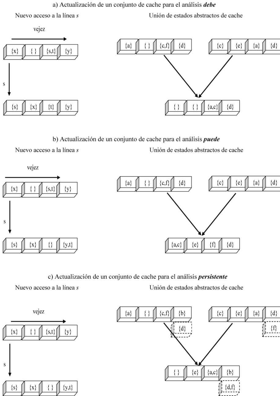
Figura 2.9: Interpretación abstracta: configuración de estados abstractos de cache.
