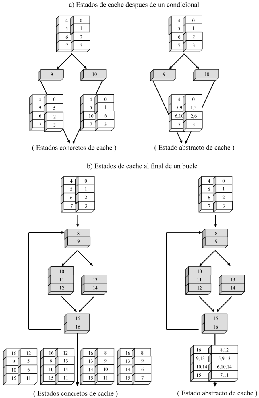
Figura 2.8: Estados concretos vs. estado abstracto conseguido mediante SCS .
