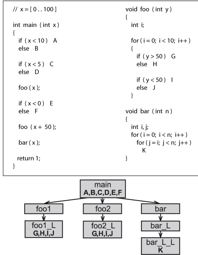
Figura 2.6: Programa con diversos caminos imposibles [75].
