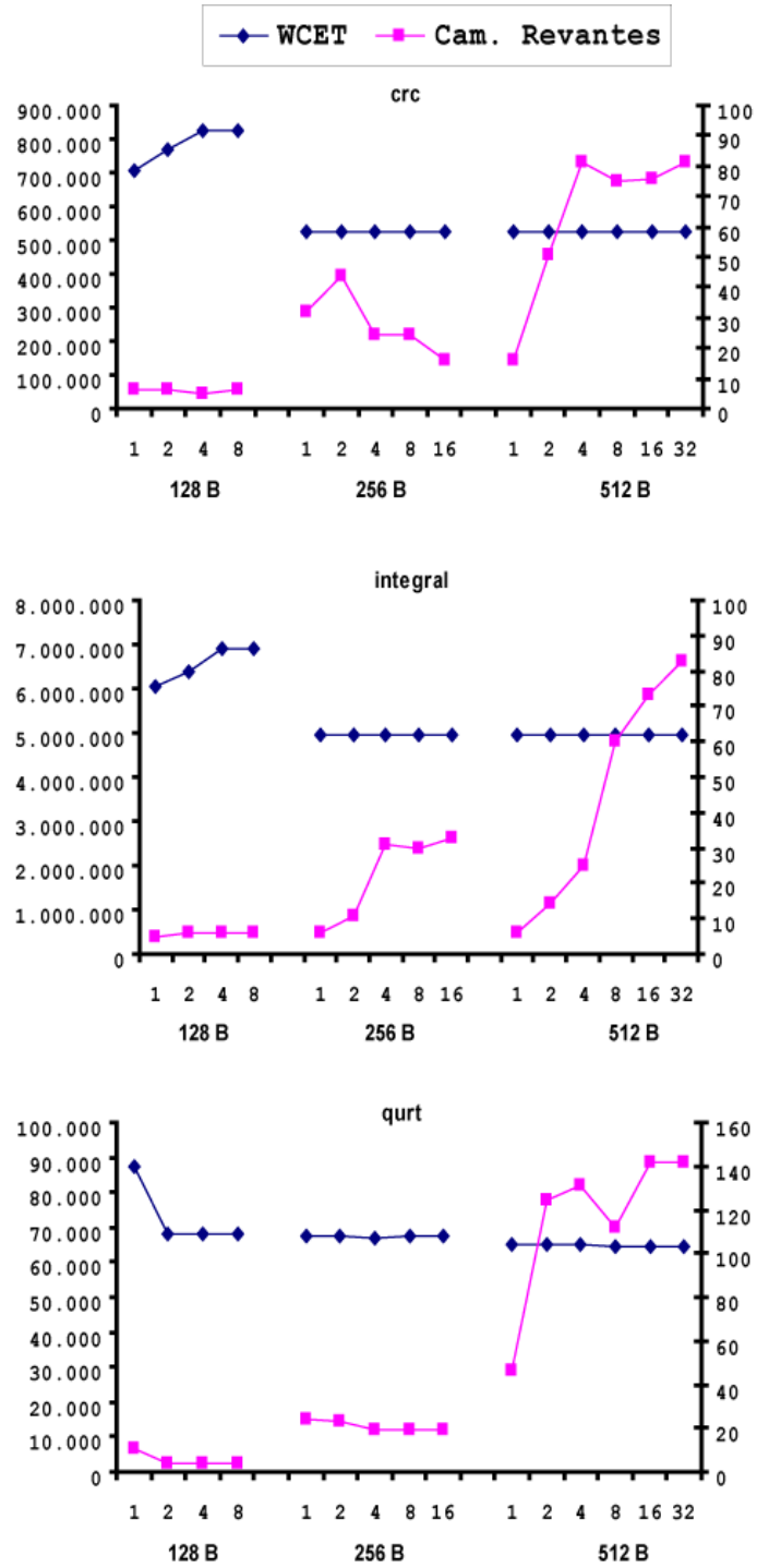
Figura 3.7: Eje Y de la izquierda: WCET. Eje Y de la derecha: caminos relevantes .
