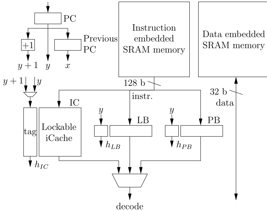
Figura 5.3: Detalle de una jerarquía de memoria para sistemas de tiempo real con prebúsqueda.
