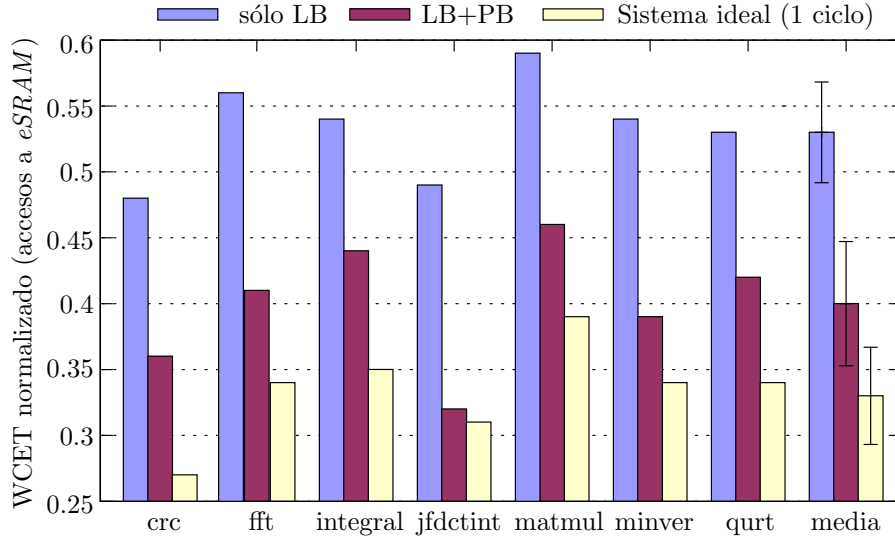
Figura 5.6: WCET de cada tarea en las 4 configuraciones consideradas.
