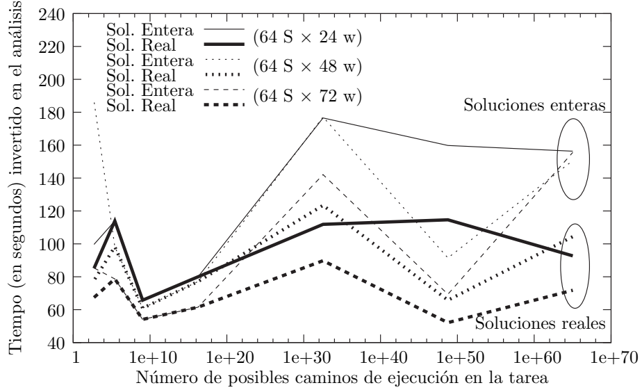
Figura 4.14: Tiempo de análisis en función del número de condicionales.
