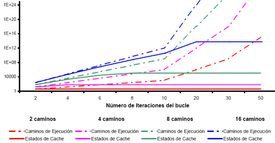
Figura 3.2: Número de caminos posibles de ejecución vs. Número de estados diferentes de cache.
