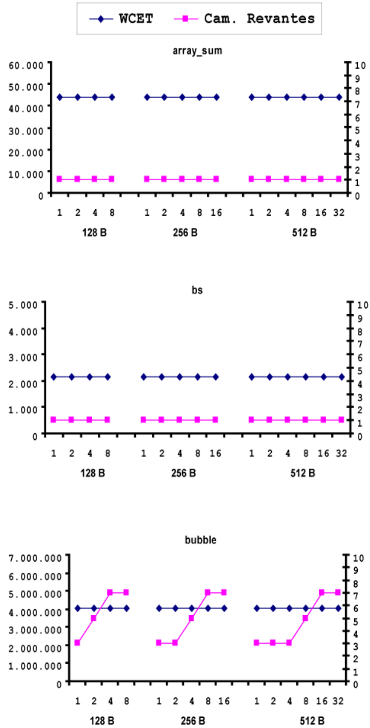
Figura 3.6: Eje Y de la izquierda: WCET. Eje Y de la derecha: caminos relevantes .
