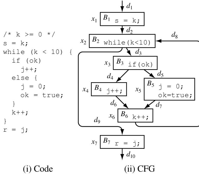
Figura 4.5: Ejemplo de programa con información funcional [107].
