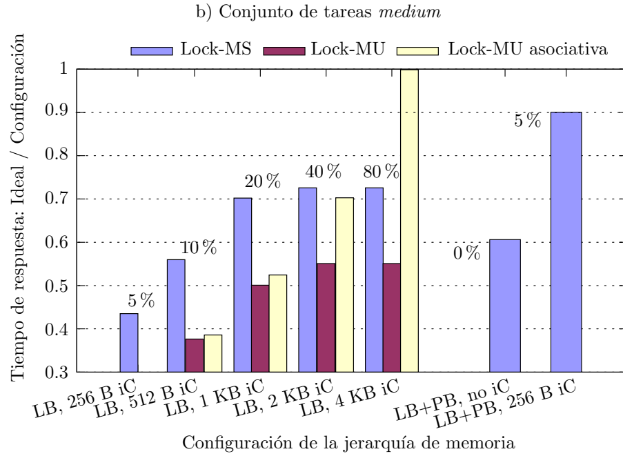
Figura 5.8: Tiempo de respuesta de la tarea de prioridad más baja, normalizado al caso ideal.
