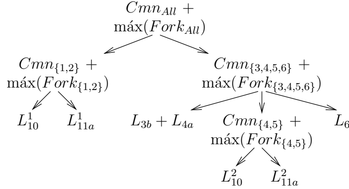
Figura 4.8: Grafo compacto de restricciones de la Figura 4.4.
