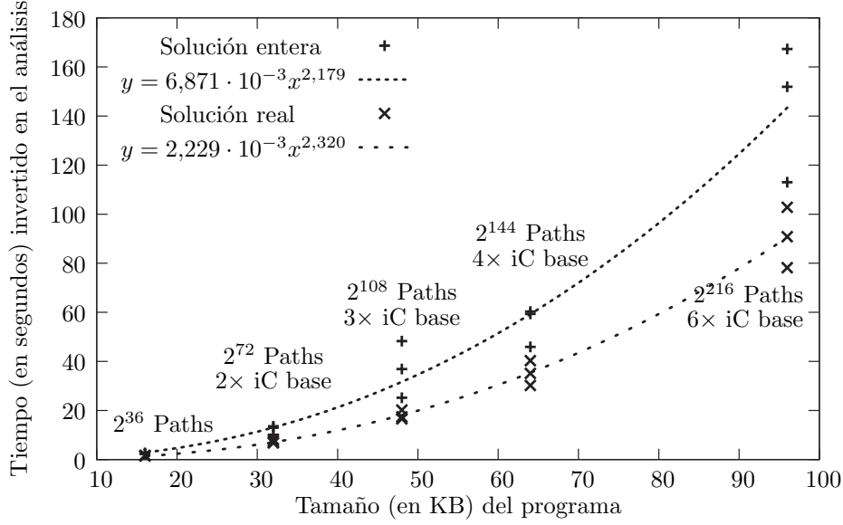
Figura 4.13: Tiempo de análisis en función de la Lockable iCache y del tamaño del programa.
