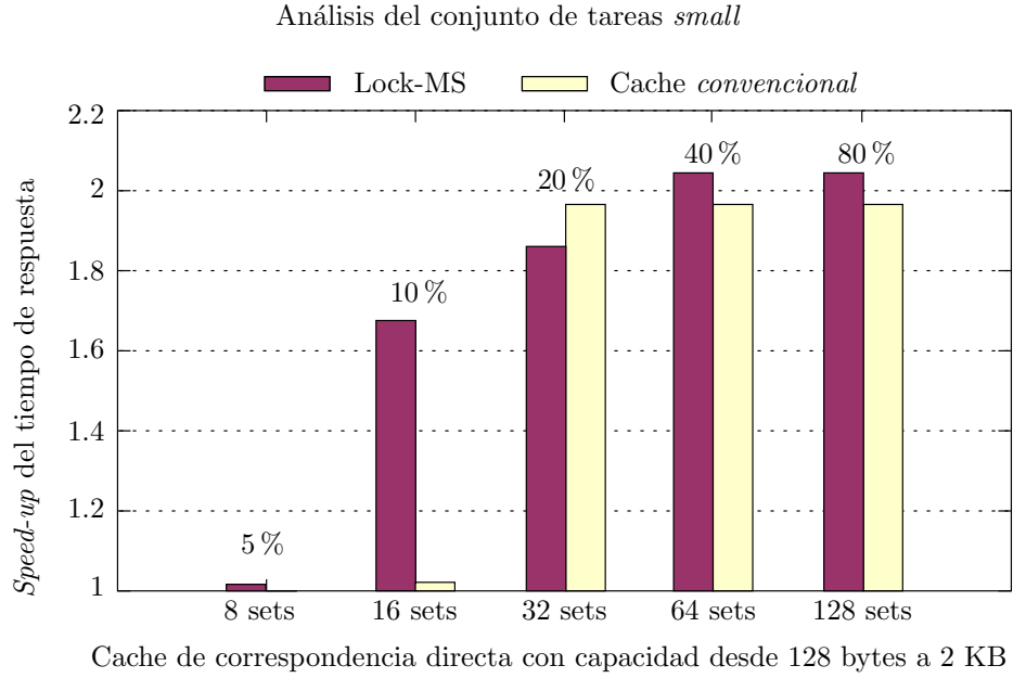
Figura 4.11: Comportamiento de Lock-MS vs. caches convencionales .
