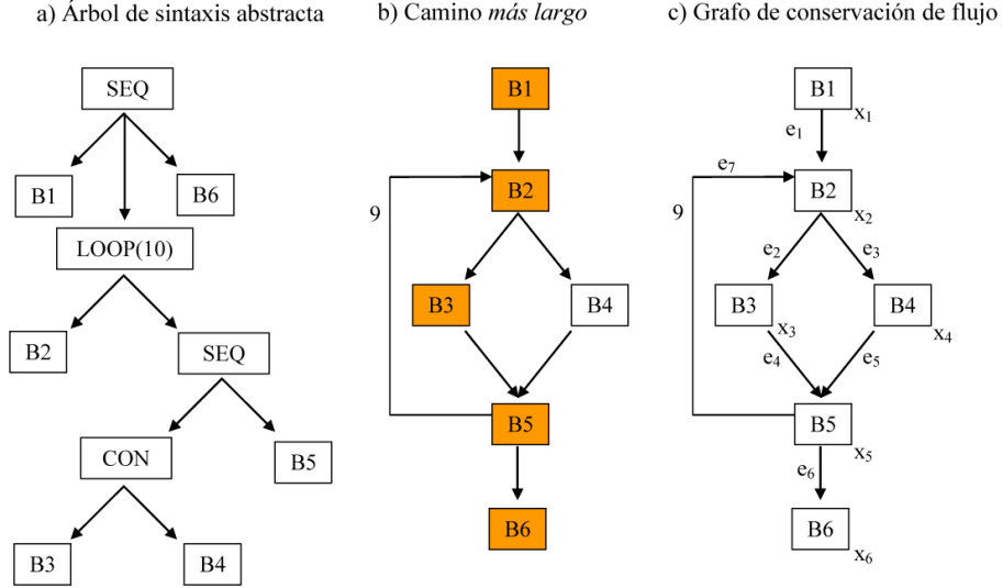
Figura 2.5: Árbol de sintaxis abstracta, grafo de flujo de control y grafo de flujo con restricciones del programa de la Figura 2.4.
