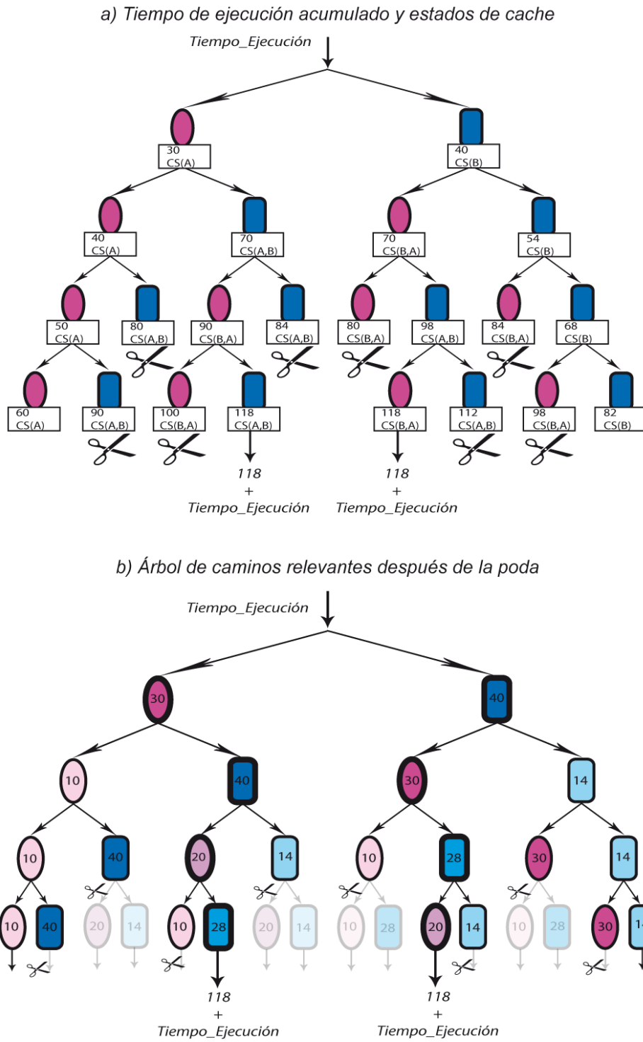
Figura 3.4: Ejemplo gráfico del cálculo preciso del WCET mediante la poda dinámica de caminos durante el análisis.
