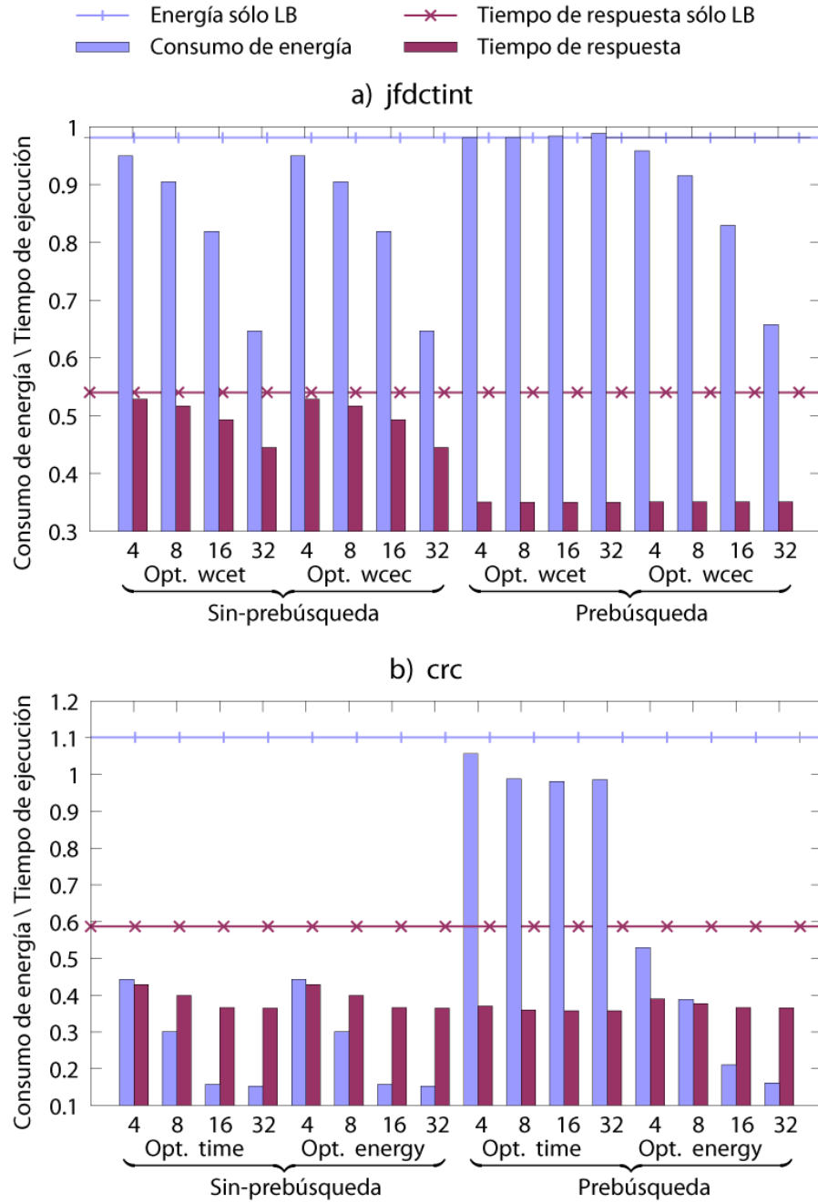
Figura 5.10: WCET y consumo de energía vs. WCEC y tiempo de ejecución de las tareas jfdctint y crc .
