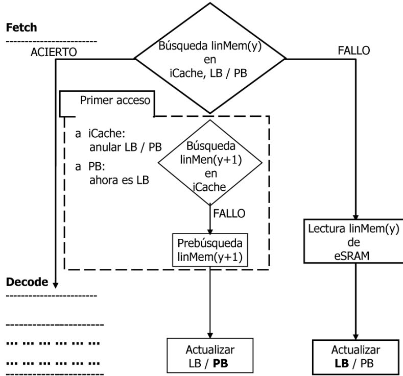
Figura 5.2: Operaciones de la prebúsqueda en la etapa de fetch cuando la iCache dispone de un puerto dual.
