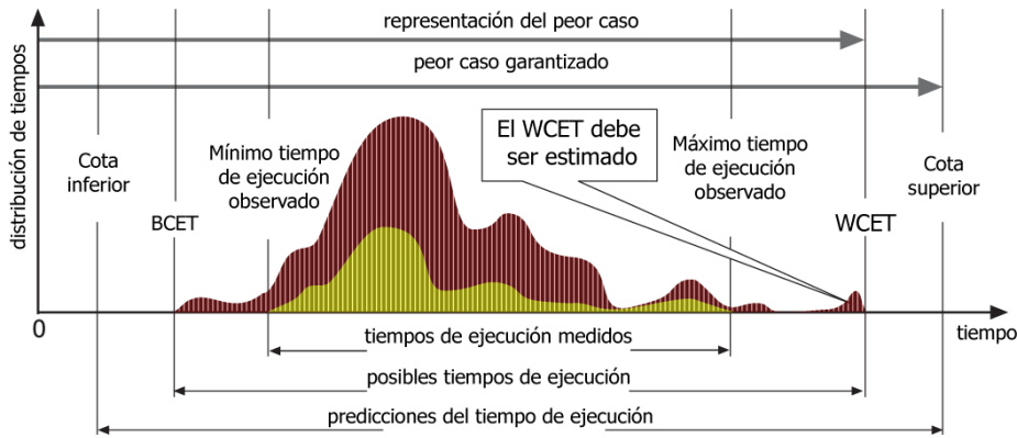
Figura 1.2: Análisis del tiempo de ejecución de una tarea [198].
