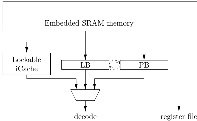
Figura 5.1: Jerarquía de memoria para sistemas de tiempo real con prebúsqueda.
