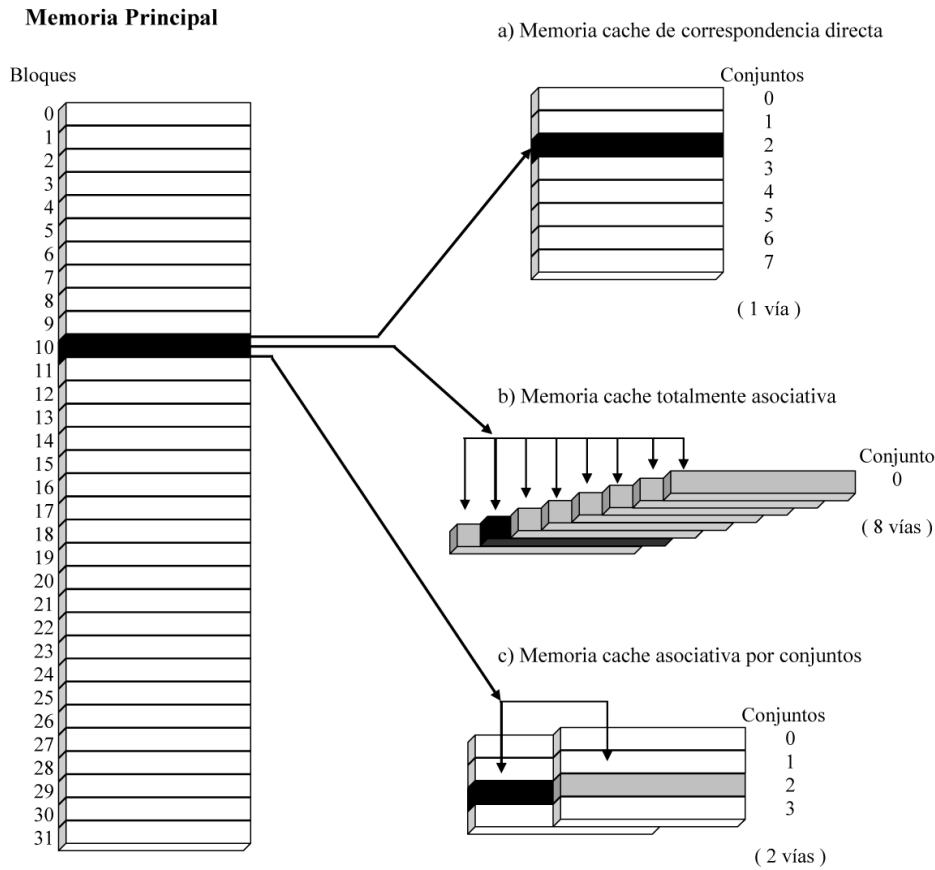
Figura 2.7: Posibles tipos de correspondencia entre bloques de memoria y líneas de cache.
