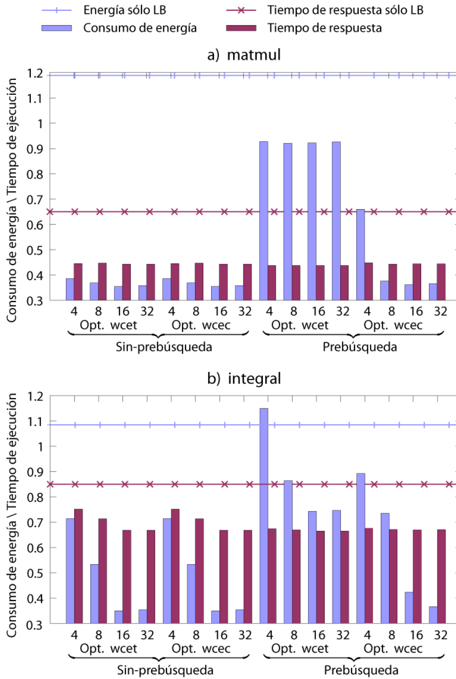
Figura 5.11: WCET y consumo de energía vs. WCEC y tiempo de ejecución de las tareas matmult e integral .
