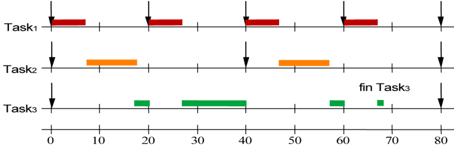
Figura 1.3: Planificación mediante RM de las nuevas tareas Task_1 , Task_2 y Task_3 .
