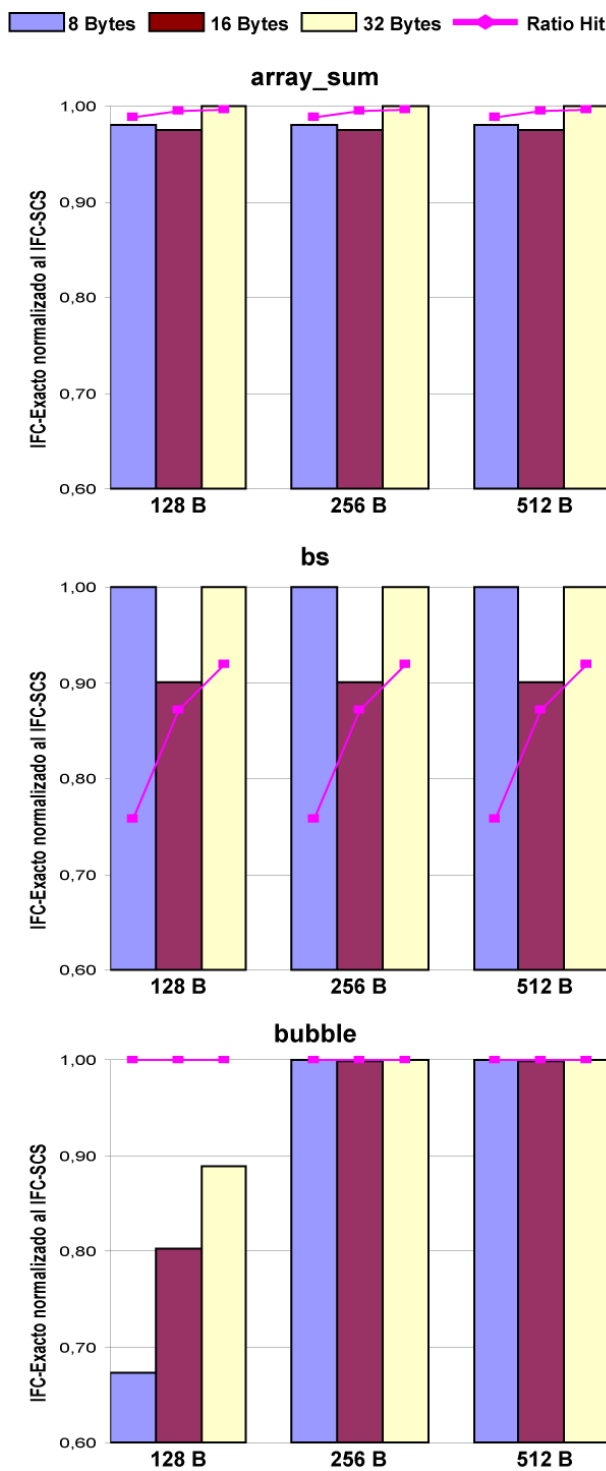
Figura 3.8: IFC exacto normalizado al IFC obtenido mediante SCS.
