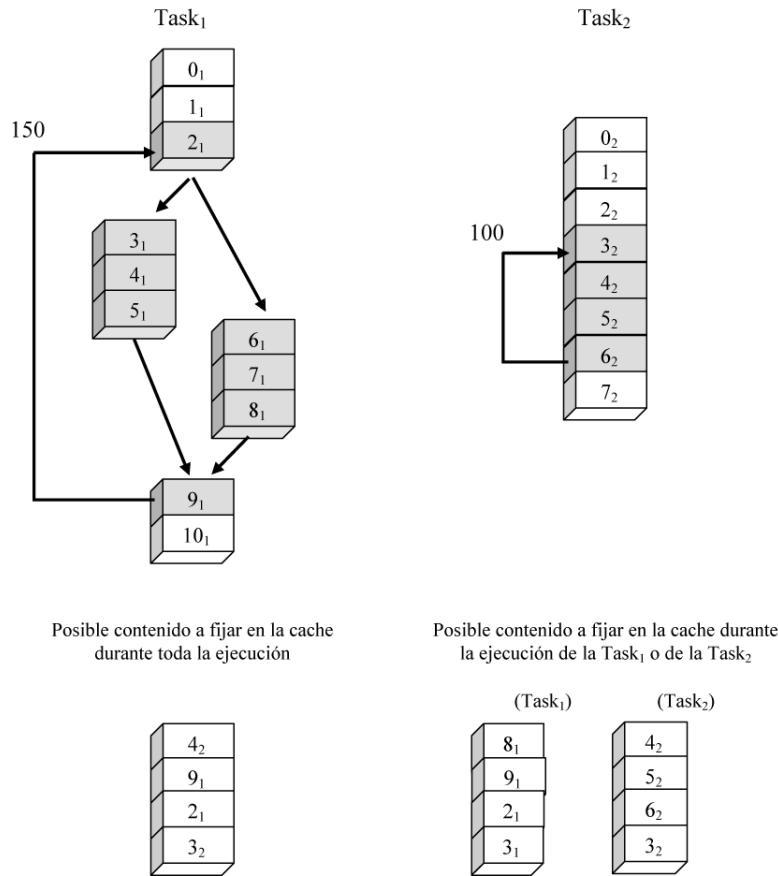
Figura 2.10: Posibles contenidos a fijar en la cache: durante toda la ejecución del sistema vs. durante la ejecución de cada tarea.
