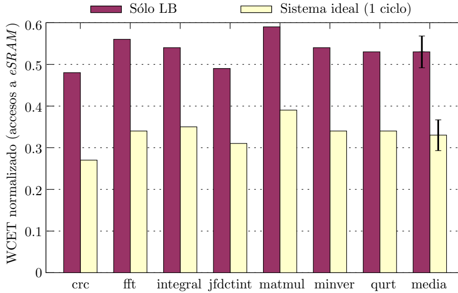
Figura 4.9: WCET de cada tarea normalizado al WCET calculado cuando se accede directamente a la eSRAM
