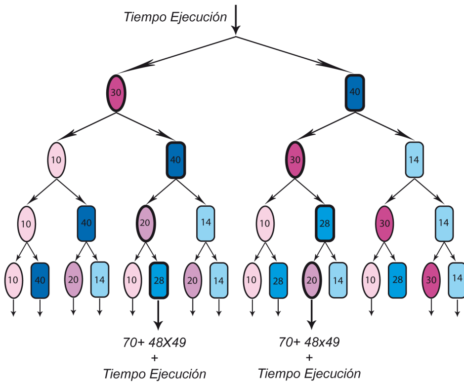
Figura 3.1: Cálculo del WCET en un bucle con un condicional.
