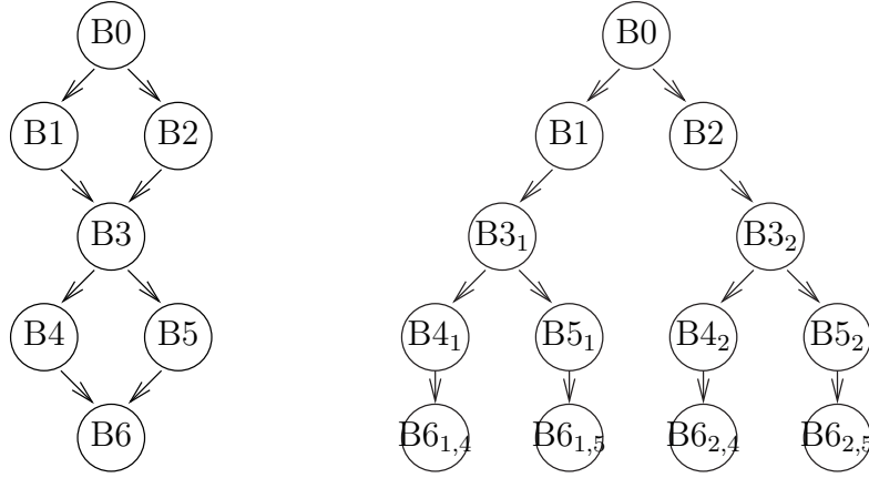
Figura 4.6: Grafo de flujo de control y explosión de los caminos de ejecución.
