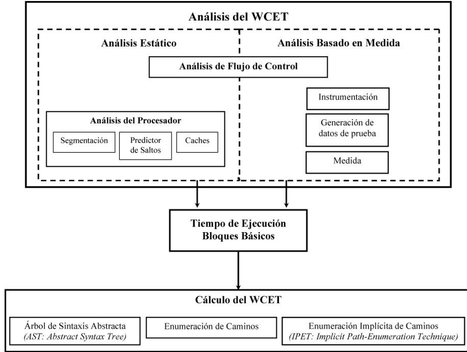
Figura 2.1: Elementos que intervienen en el análisis y cálculo del WCET.
