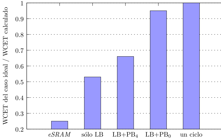
Figura 5.9: Efecto de la penalización de prebúsqueda en el WCET sin caches.
