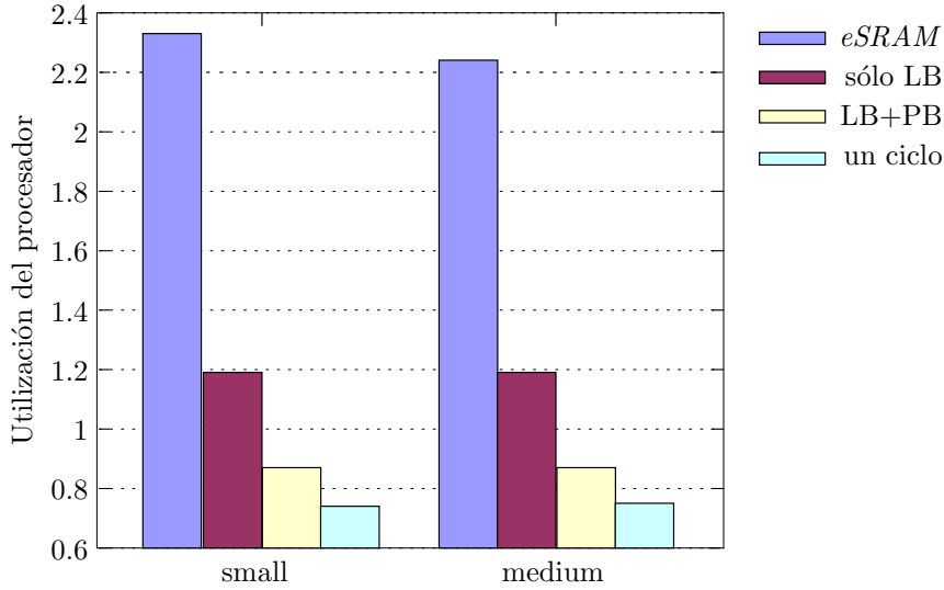
Figura 5.7: Utilización del procesador para los conjuntos de tareas small y medium .
