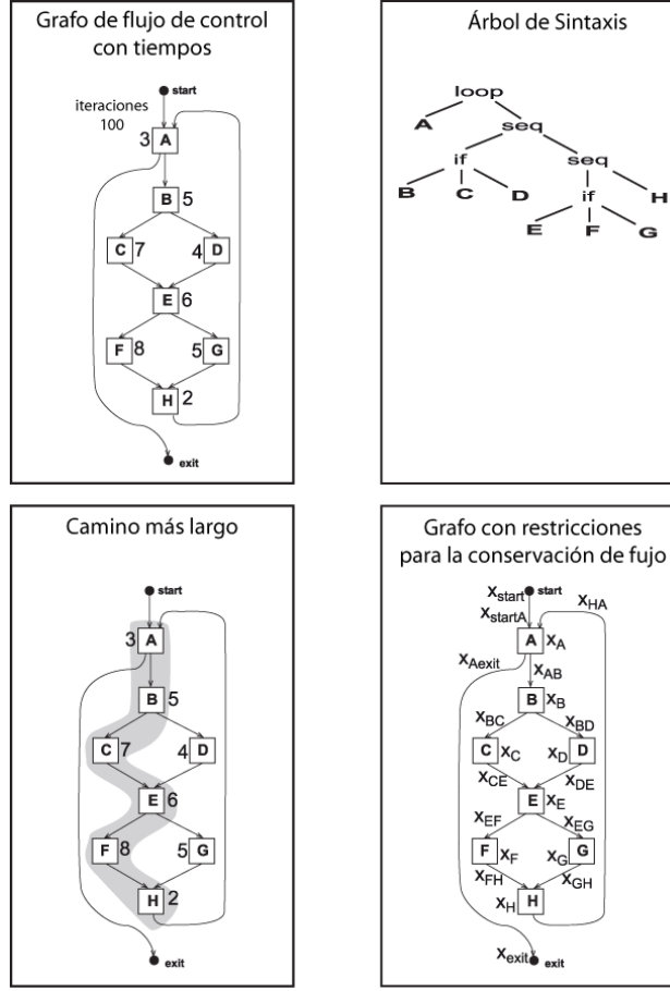
Figura 2.2: Grafo de flujo de control, árbol de sintaxis abstracta, camino más largo y grafo de flujo de control con restricciones [198].
