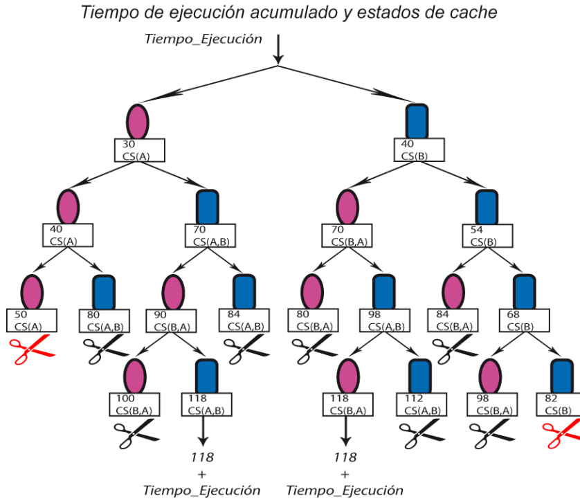
Figura 3.5: Cálculo preciso del WCET cuando el coste de cargar la caché es 50.
