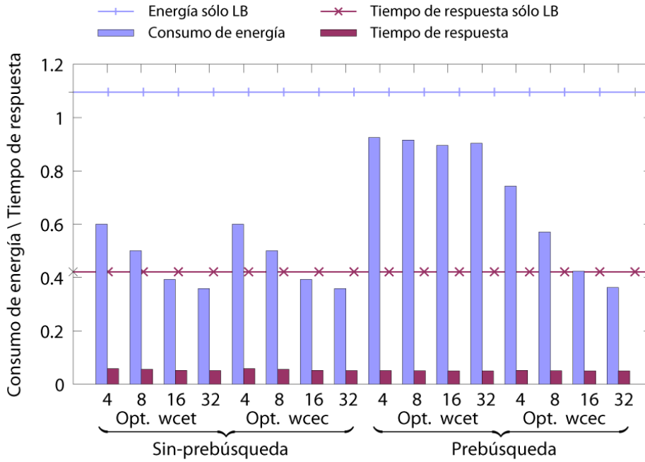
Figura 5.12: Tiempo de respuesta y consumo de energía vs. WCEC y tiempo de ejecución del conjunto de tareas small .
