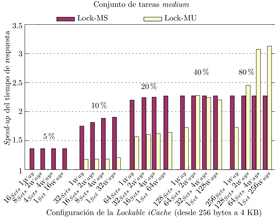
Figura 4.10: Speed-up del tiempo de respuesta para los conjuntos de tareas small y medium .
