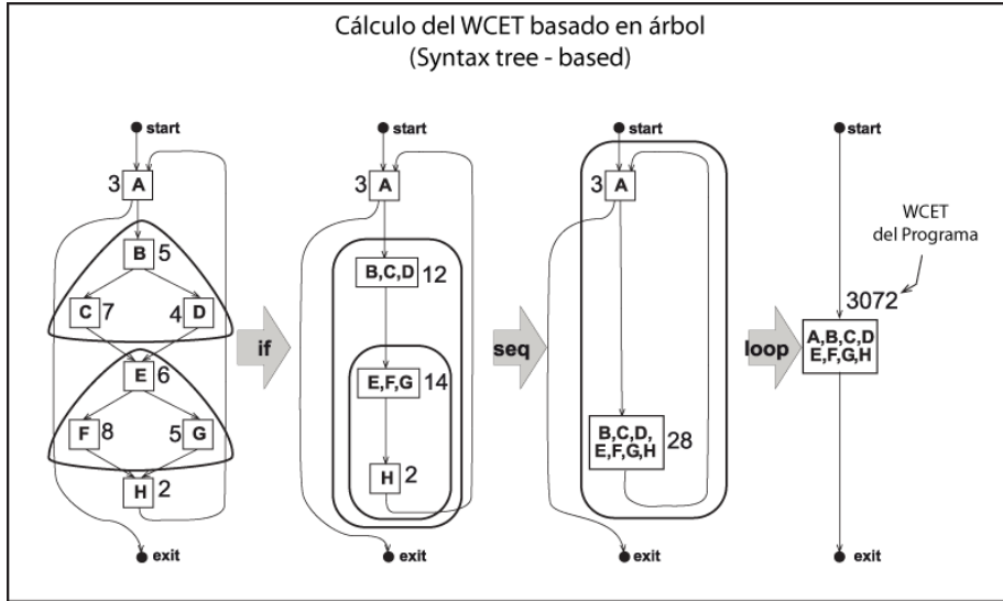
Figura 2.3: Esquema que sigue el cálculo del WCET basado en AST [198].
