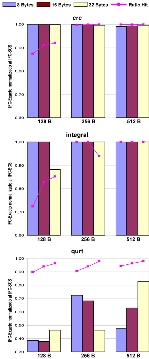
Figura 3.9: IFC exacto normalizado al IFC obtenido mediante SCS.
