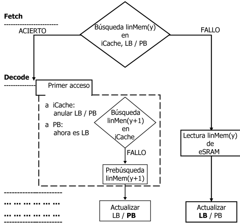
Figura 5.4: Operaciones de la prebúsqueda en las etapas de fetch y decode cuando la iCache sólo tiene un puerto.
