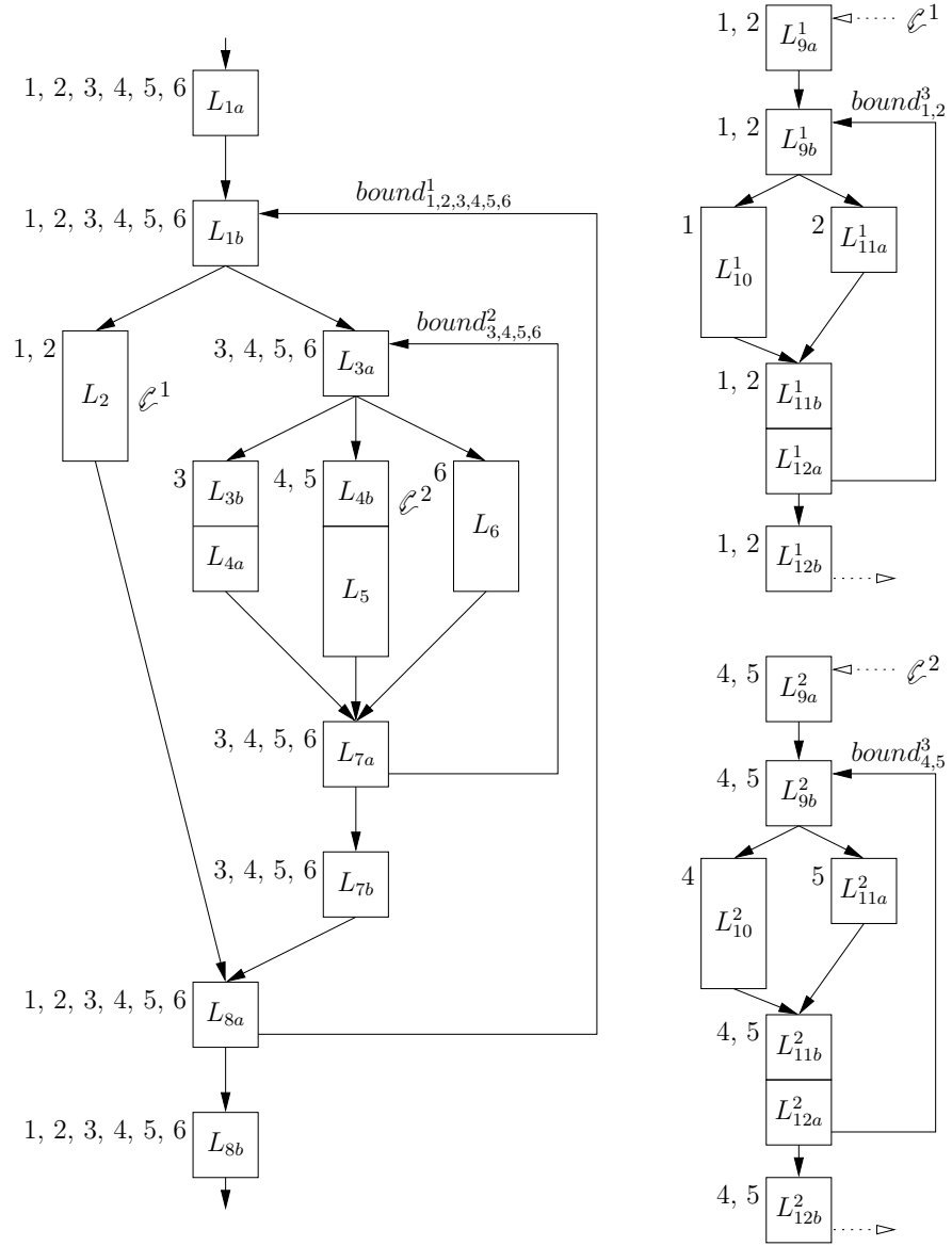
Figura 4.4: Modelado del flujo de control donde: a) las líneas de memoria divididas se han identificado de forma única, b) se han introducido las instancias a la función, c) se han anotado los caminos a los que pertenece cada bloque básico.
