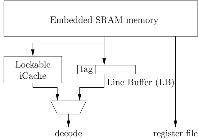
Figura 4.1: Jerarquía de memoria para instrucciones en un sistema de tiempo real.
