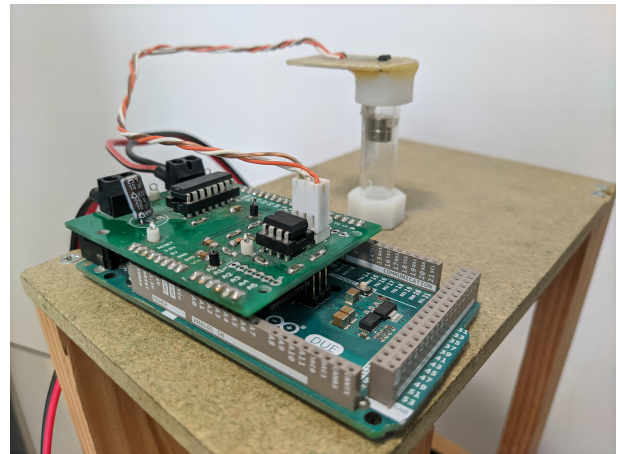
Figura 2: Componentes electrónicos del sistema. La base es la placa de desarrollo Arduino Due. Encima, la PCB que aloja las etapas electrónicas de sensado y de potencia. De fondo se puede ver el imán levitando en el interior del tubo.
