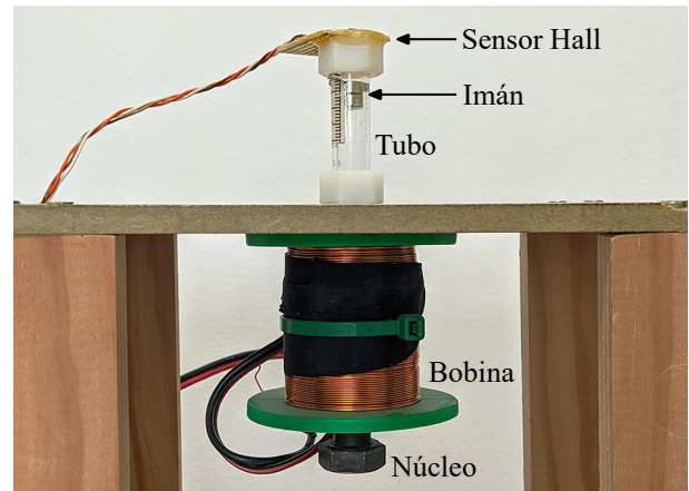
Figura 1: Levitador magnético. El imán levita en el interior de un tubo transparente de metacrilato. El movimiento de levitación se puede controlar actuando sobre el electroimán formado por la bobina y el núcleo ferromagnético.
