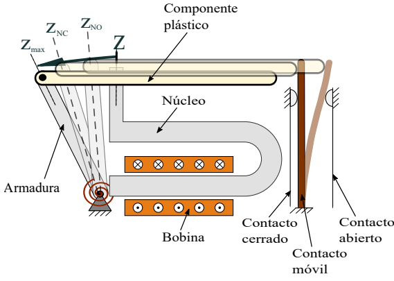
Figura 1: Representación esquemática del dispositivo de trabajo. Posiciones: z_{\max} (máxima), z_{NC} (el contacto móvil despega del contacto cerrado) y z_{NO} (el contacto móvil contacta con el contacto abierto).
